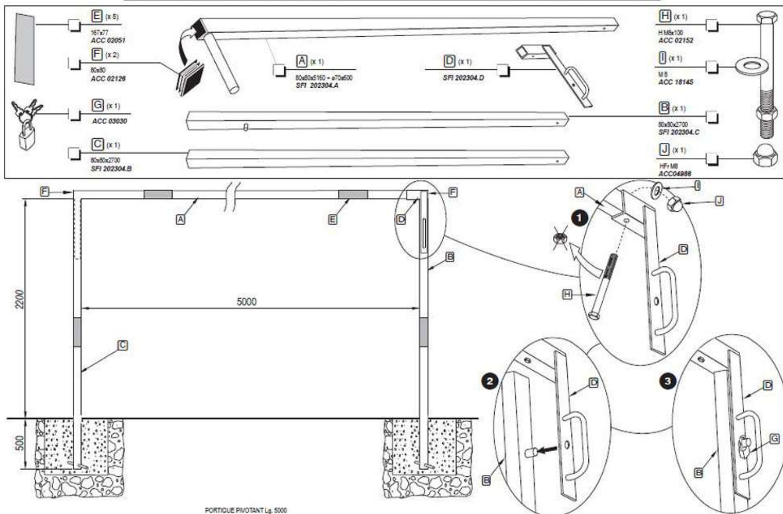
PORTIQUE PIVOTANT Lg 5000
